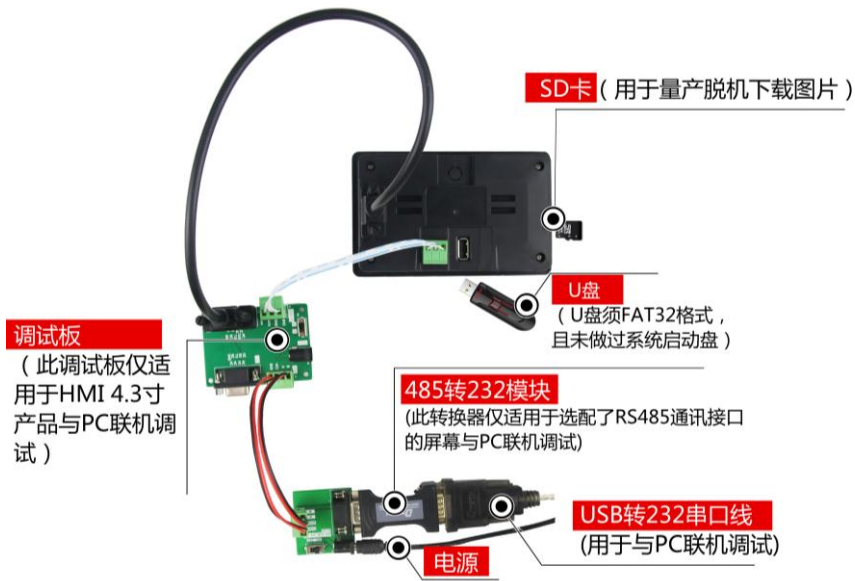
图 1-3 RS485 调试图
