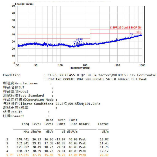
图 6-6 RE 测试垂直方向
