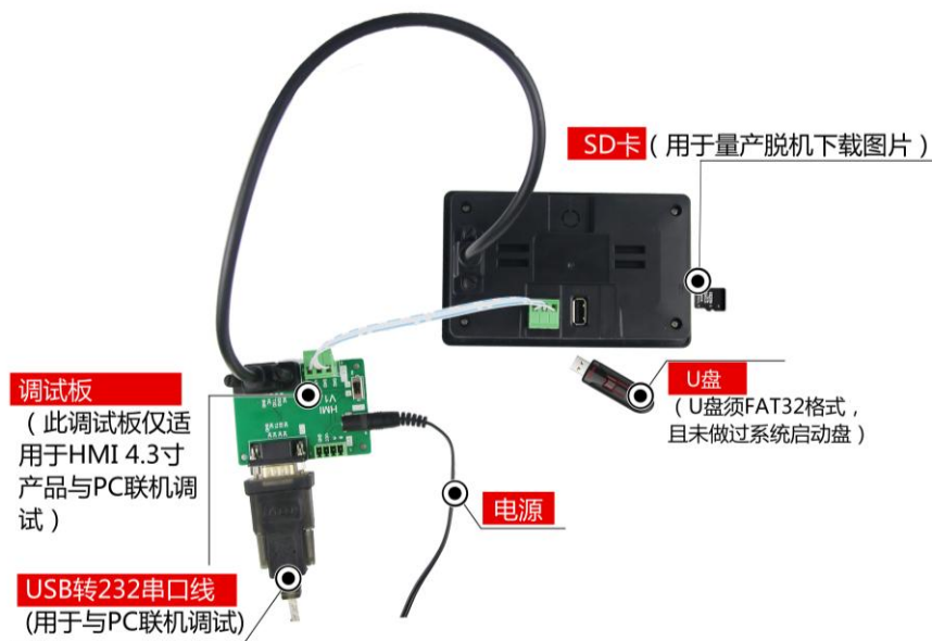
图 1-4 RS232 调试图
