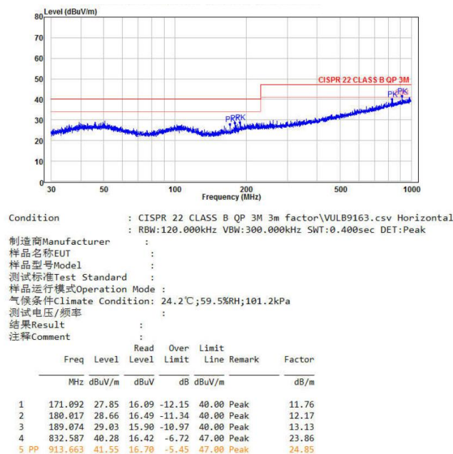
图 6-5 RE 测试水平方向
